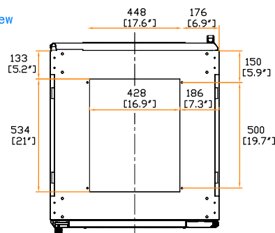
Front door
