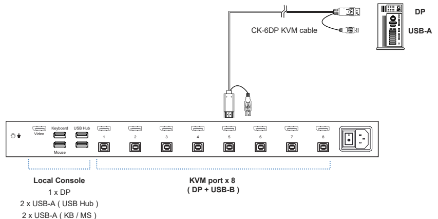
CK-6DP DP KVM cable, 6 ft 4K 60Hz
